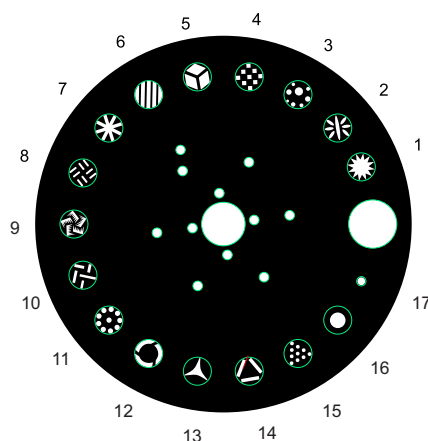
Statisches Goborad/ static gobo wheel
