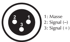
DMX-Ausgang XLR-Einbaubuchse:
