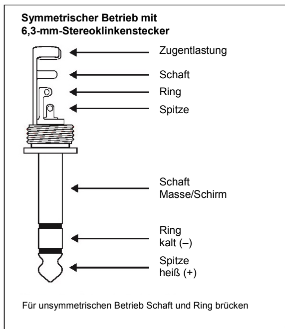
Abb. 5.4 6,3-mm-Stereoklinkenstecker
