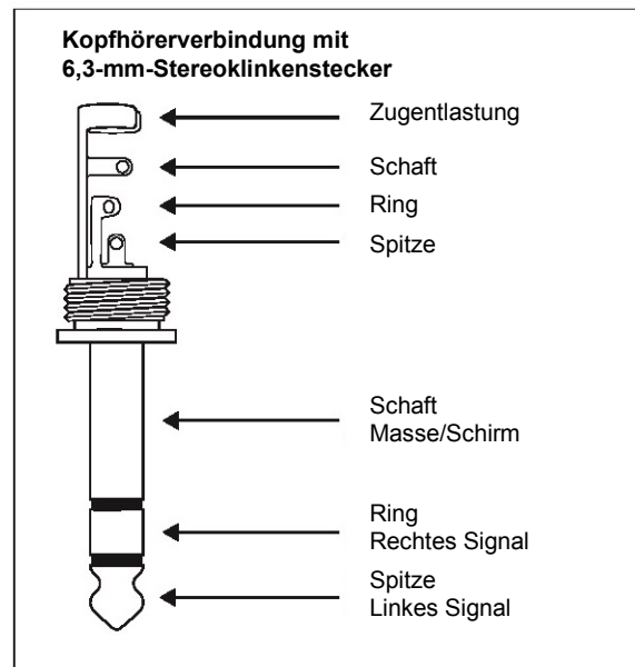
Abb. 5.6 Kopfhörer-Stereoklinkenstecker
