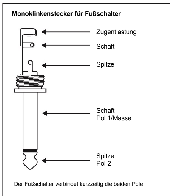
Abb. 5.1 Fußschalter
