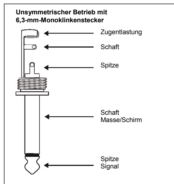
Abb. 5.3 6,3-mm-Monoklinkenstecker
