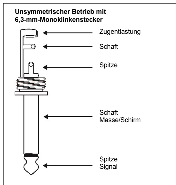
Abb. 5.3 6,3-mm-Monoklinkenstecker
