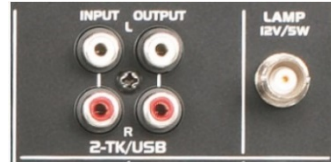
Abb. 4.15 Cinch-Anschlüsse und Lampenanschluss
