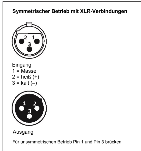
Abb. 5.2 XLR-Verbindungen
