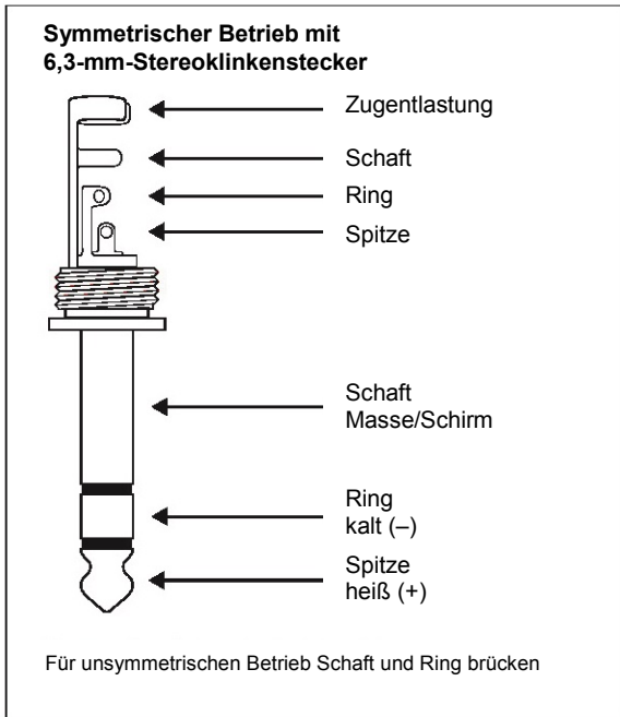
Abb. 5.4 6,3-mm-Stereoklinkenstecker
