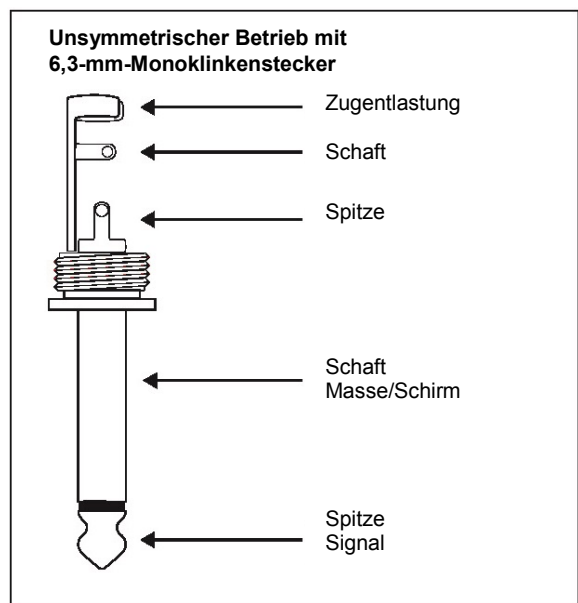
Abb. 5.3 6,3-mm-Monoklinkenstecker
