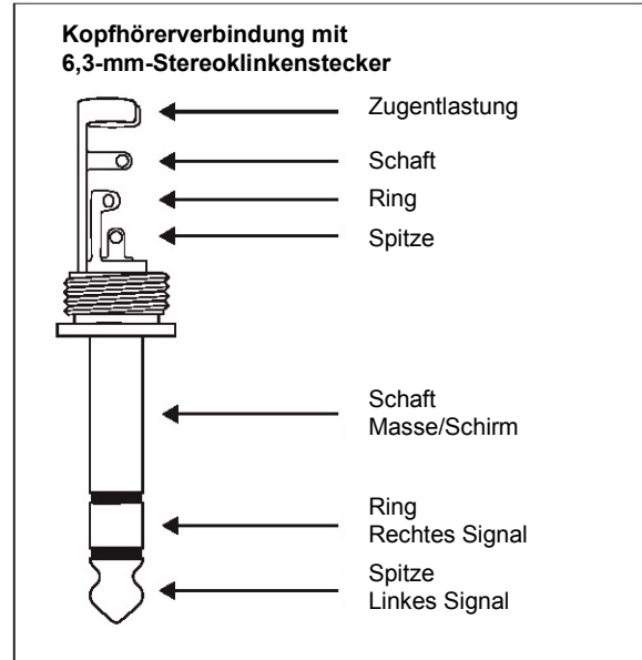
Abb. 5.6 Kopfhörer-Stereoklinkenstecker
