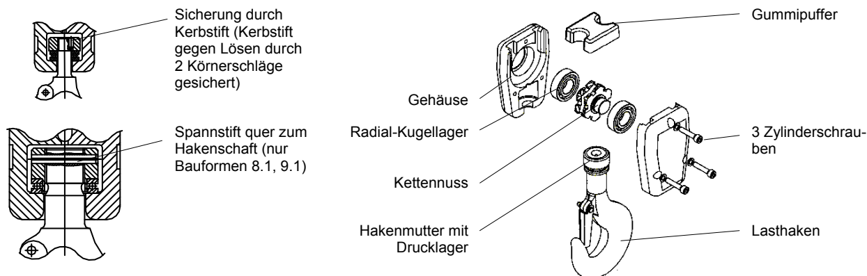
Bild 28 Aufbau der Hakenflasche
