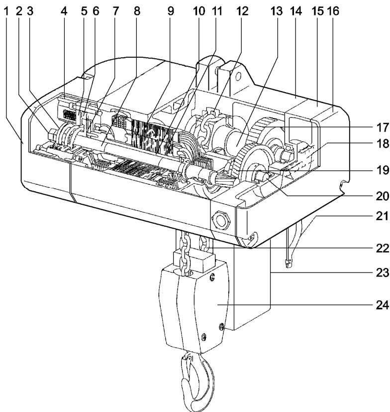
Bild 2 Schnittbild
