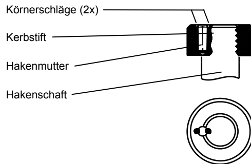
Bild 46 Hakenmuttersicherung
