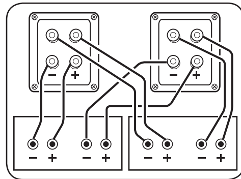
Bi-Amping
