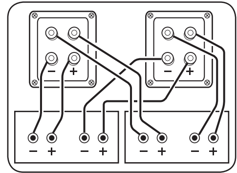
Bi-Amping
