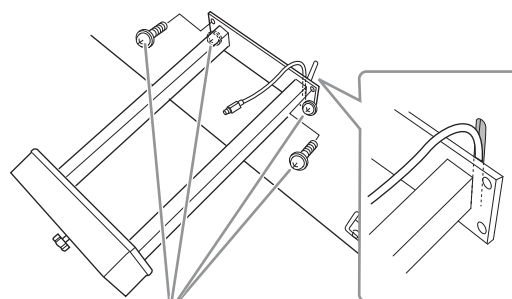
Befestigungsschrauben (6 x 20 mm)
