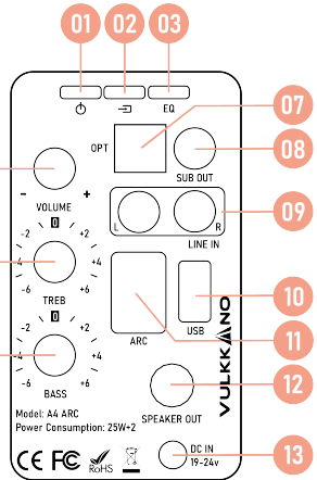
Aktiv-Lautsprecher
