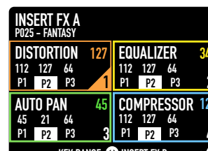
Insert FX-Einstellungen
