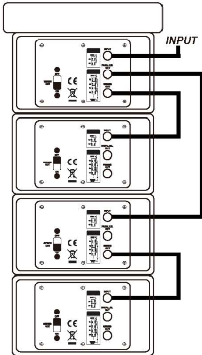
4 Module.array (8.ohms)
