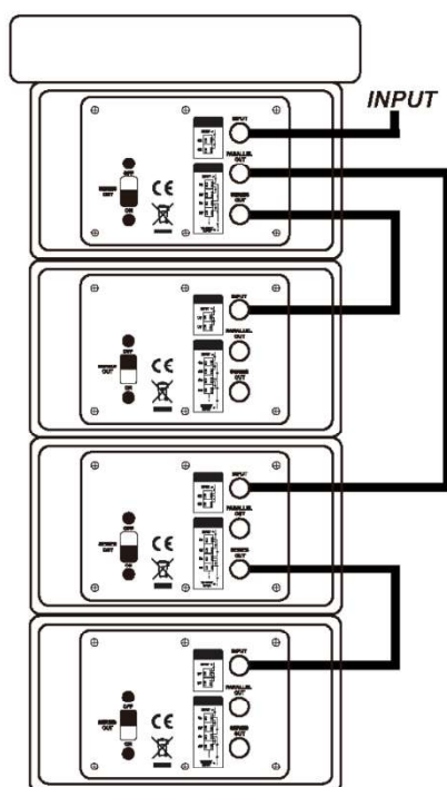
4 Module.array (8.ohms)
