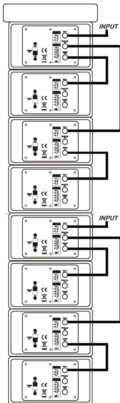
8 Module.array (4.ohms)
