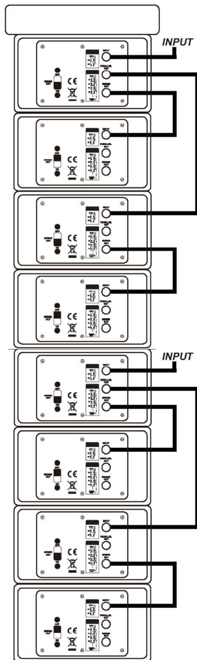
8 Module.array (4.ohms)
